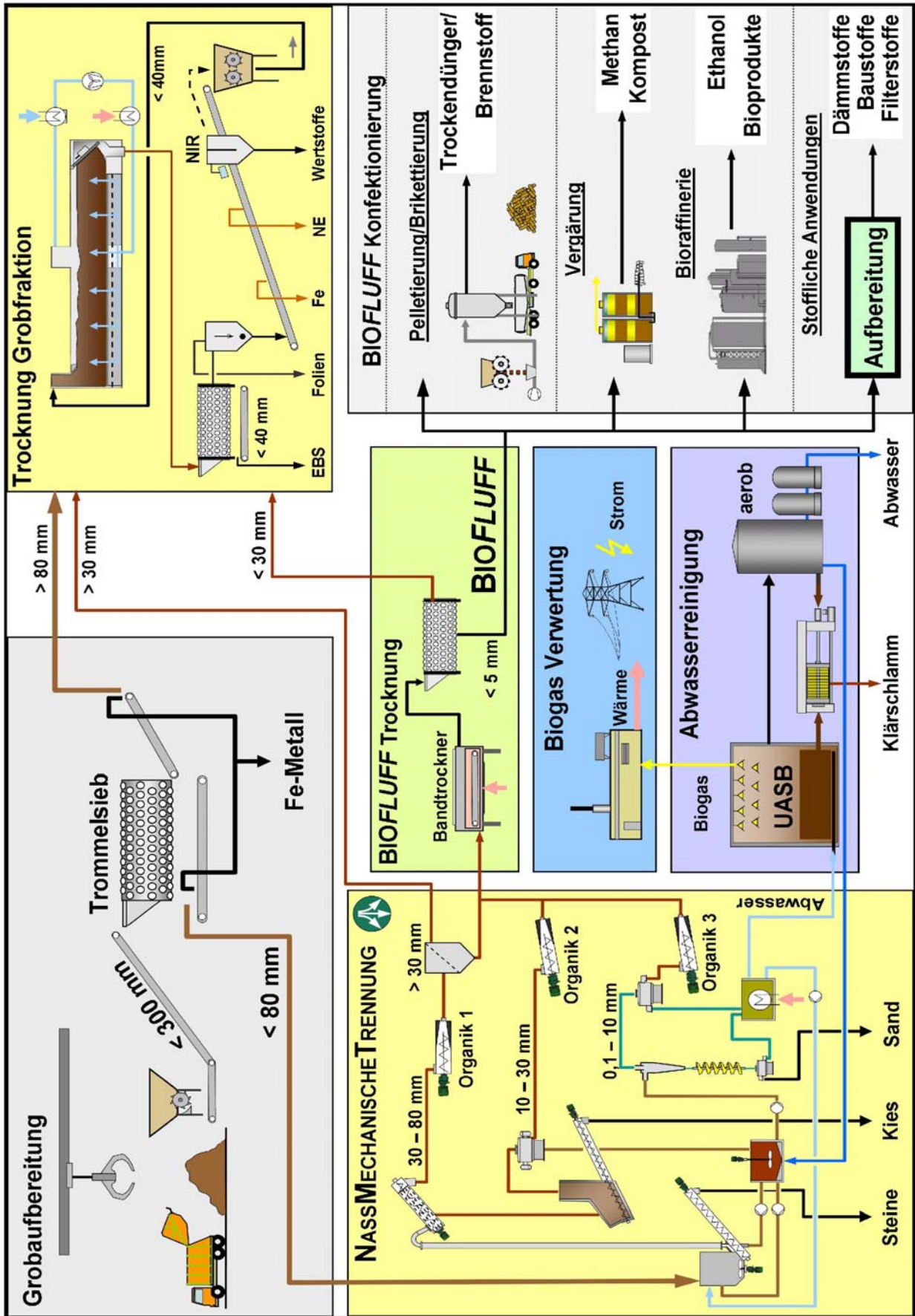
Abbildung 3: Verfahrensschema gesamt
