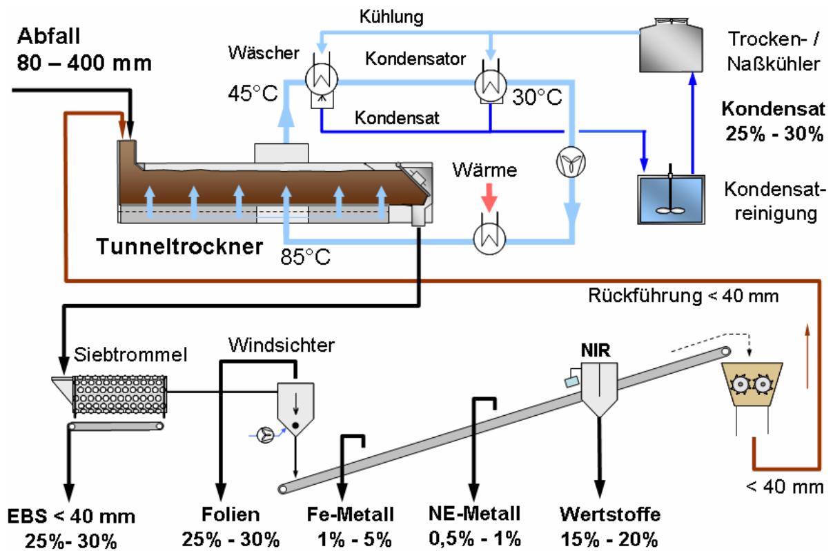
Abbildung 1: Verfahrensfliessbild Tunneltrockner mit Aufbereitung
